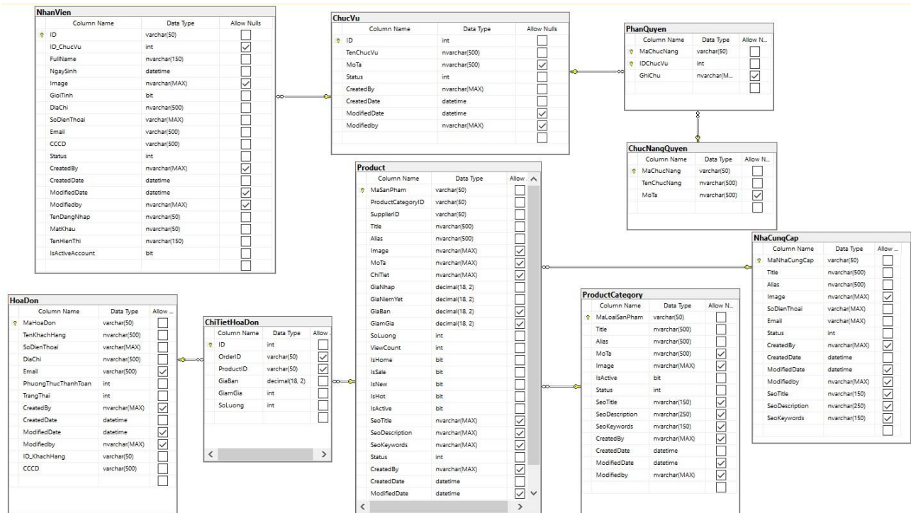
Hình 3.1. Sơ đồ logic được thiết kế bằng SQL Server
